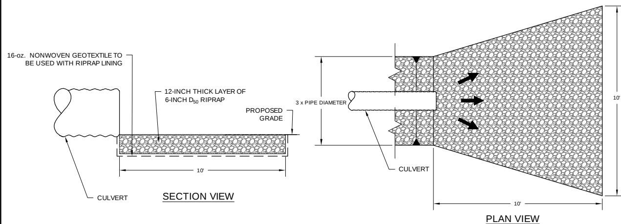
3 RIPRAP APRON DETAIL
