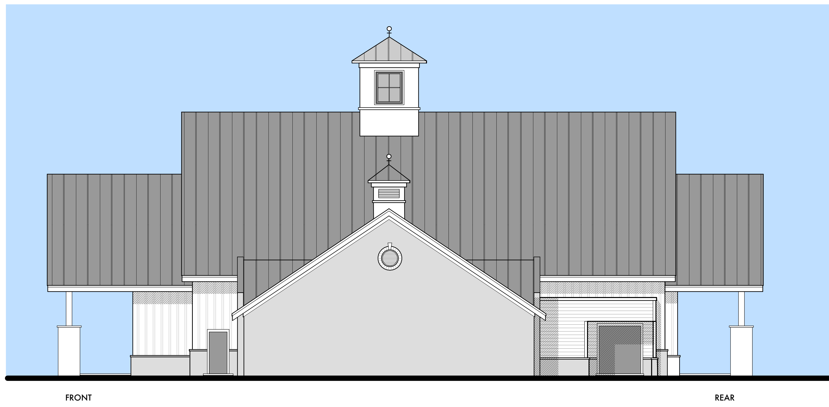
1 RIGHT SIDE ELEVATION Scale: 1/8" = 1'-0"
